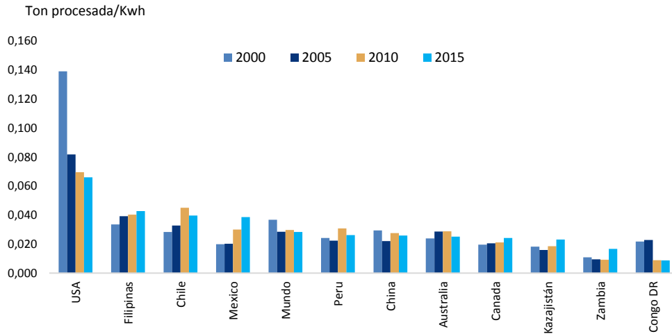
Fig. 20: Evolución de ton/kwh procesada en minas medianas de cobre a nivel mundial entre 2000-2015
