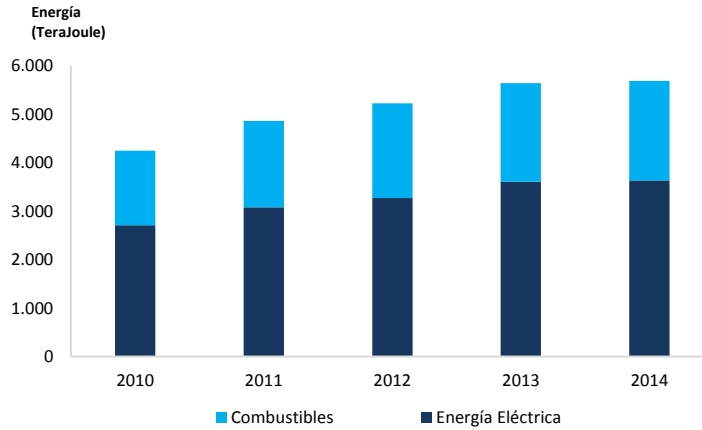
Fig. 14: Evolución del consumo de energía de las empresas de la mediana minería del cobre encuestadas
