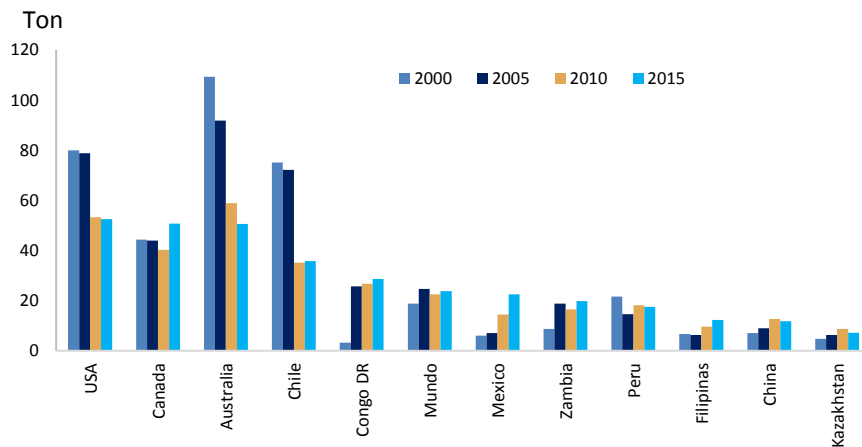
Fig. 21: Evolución de ton cobre/trabajador en minas medianas de cobre a nivel mundial entre 2000-2015
