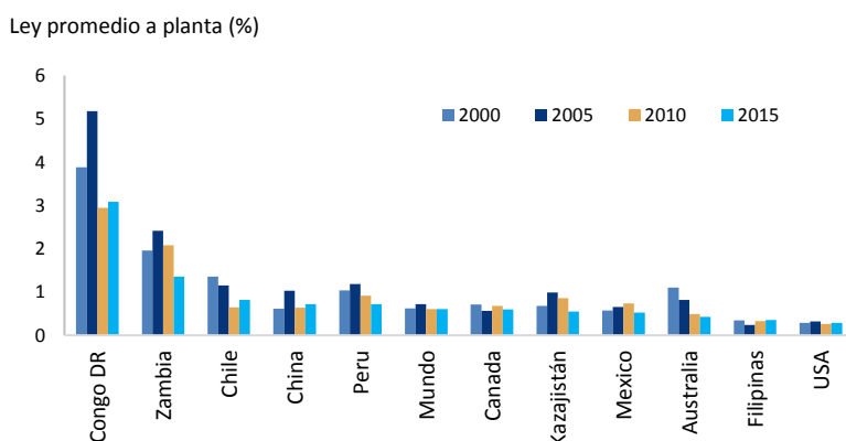
Fig. 22: Evolución de ley promedio a planta en minas medianas de cobre a nivel mundial entre 2000-2015
