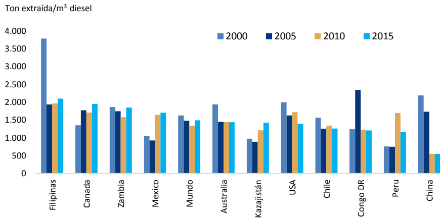
Fig. 19: Evolución de ton extraída/m 3 diesel en minas medianas de cobre a nivel mundial entre 2000-2015
