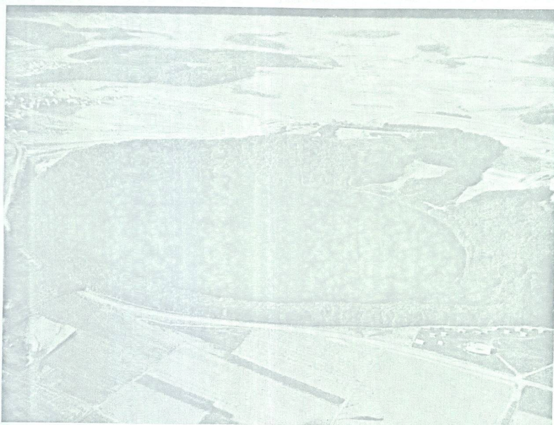
FIG. 8 - Pulvermaar. (Photo C. D. Ollier).
