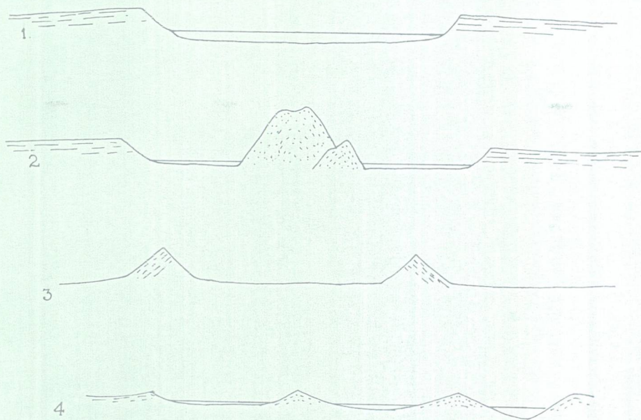
FIG. 13 - Types of maars. 1. Pulvermaar - 2. Zuni - 3. Koki - 4. Red Rock.
