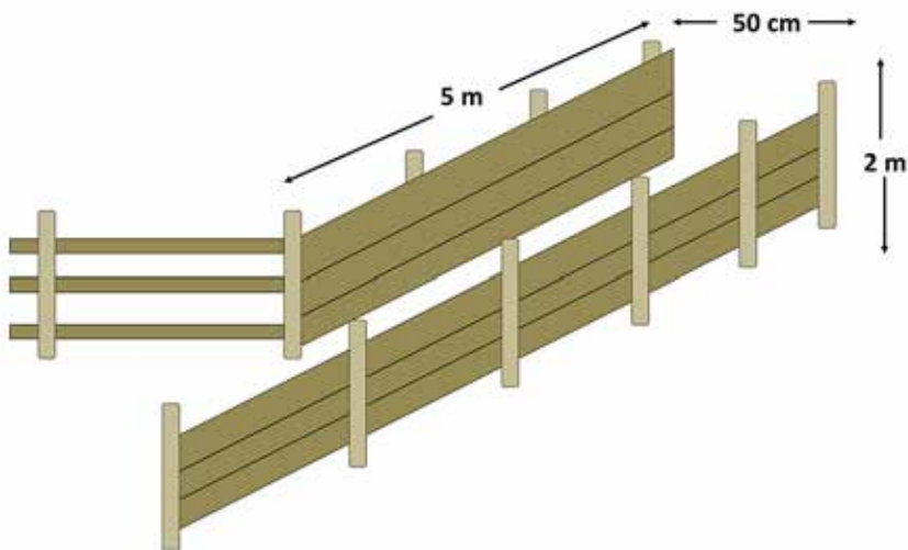
Figura 8.14. Manga con embudo para ovinos.
