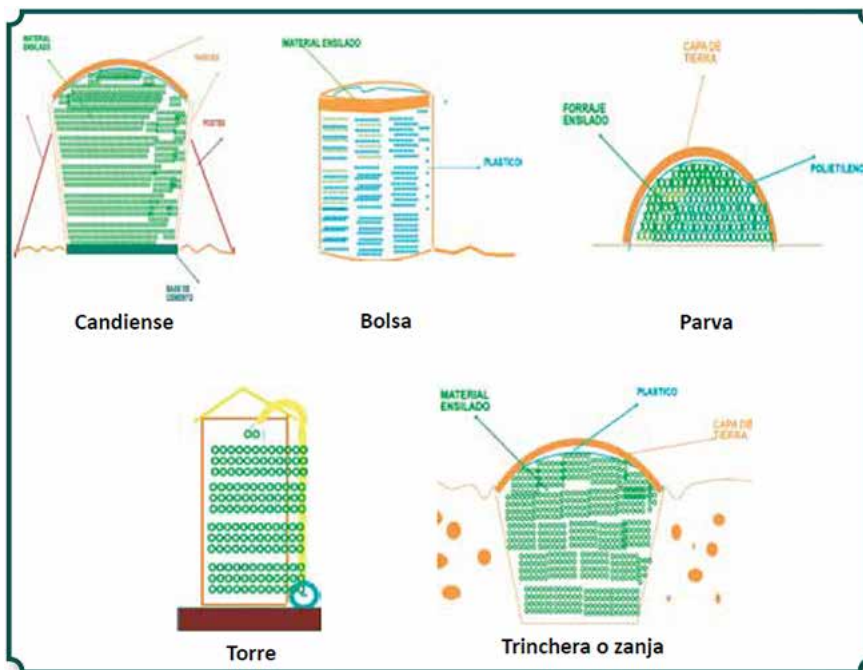
Figura 3.1. Diferentes tipos de silo.
