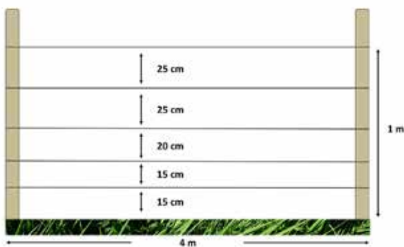
Figura 8.3. Cerco de alambre liso para ovinos.
