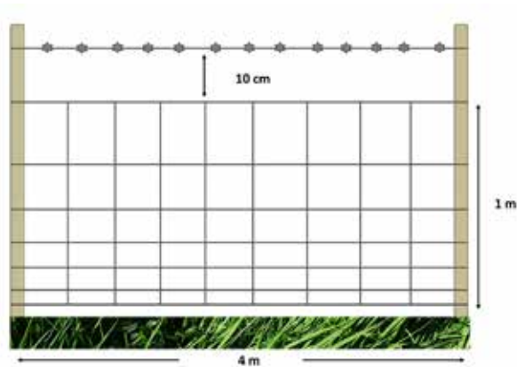
Figura 8.1. Cerco perimetral de malla ursum para ovinos.
