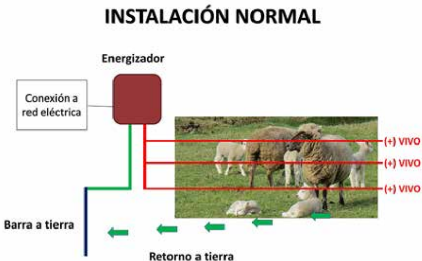
Figura 8.5. Generador y cable a tierra de un sistema de cerco eléctrico.
