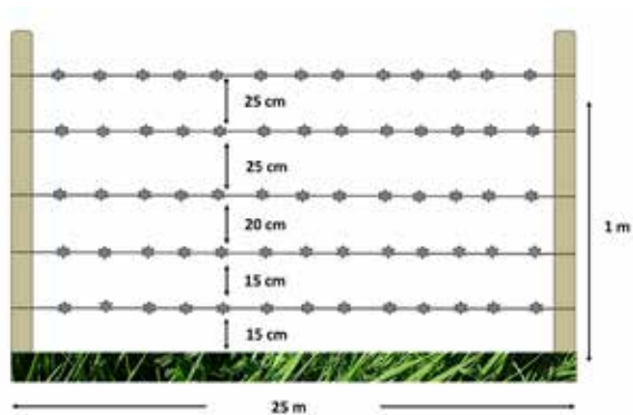
Figura 8.2. Cerco de alambre de púas para ovinos
