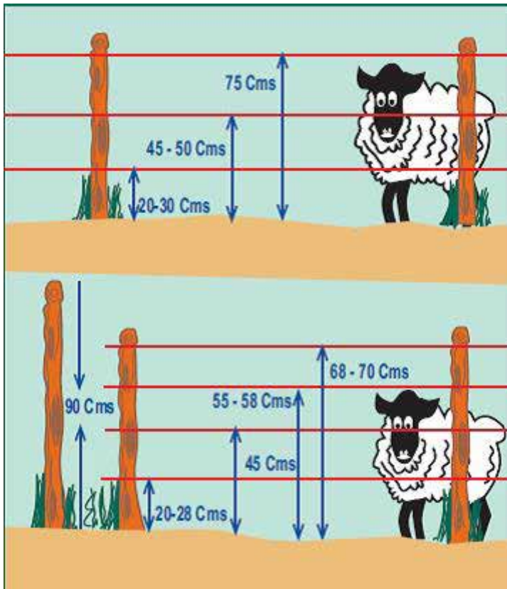
Figura 8.4. Cerco eléctrico para ovinos.
