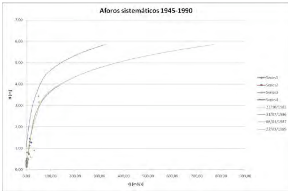
Ilustración 50: Aforos sistemáticos (series) y curvas de descarga 1945-1990 – Cauquenes en el Arrayan
