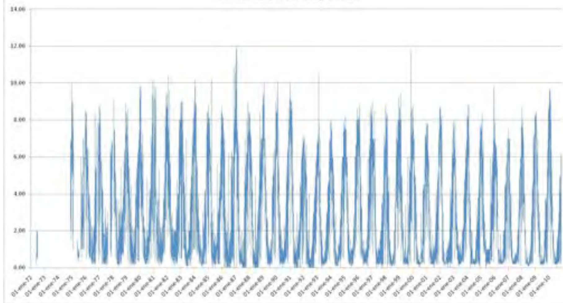
DIGUA EMBALSE - Evaporación
