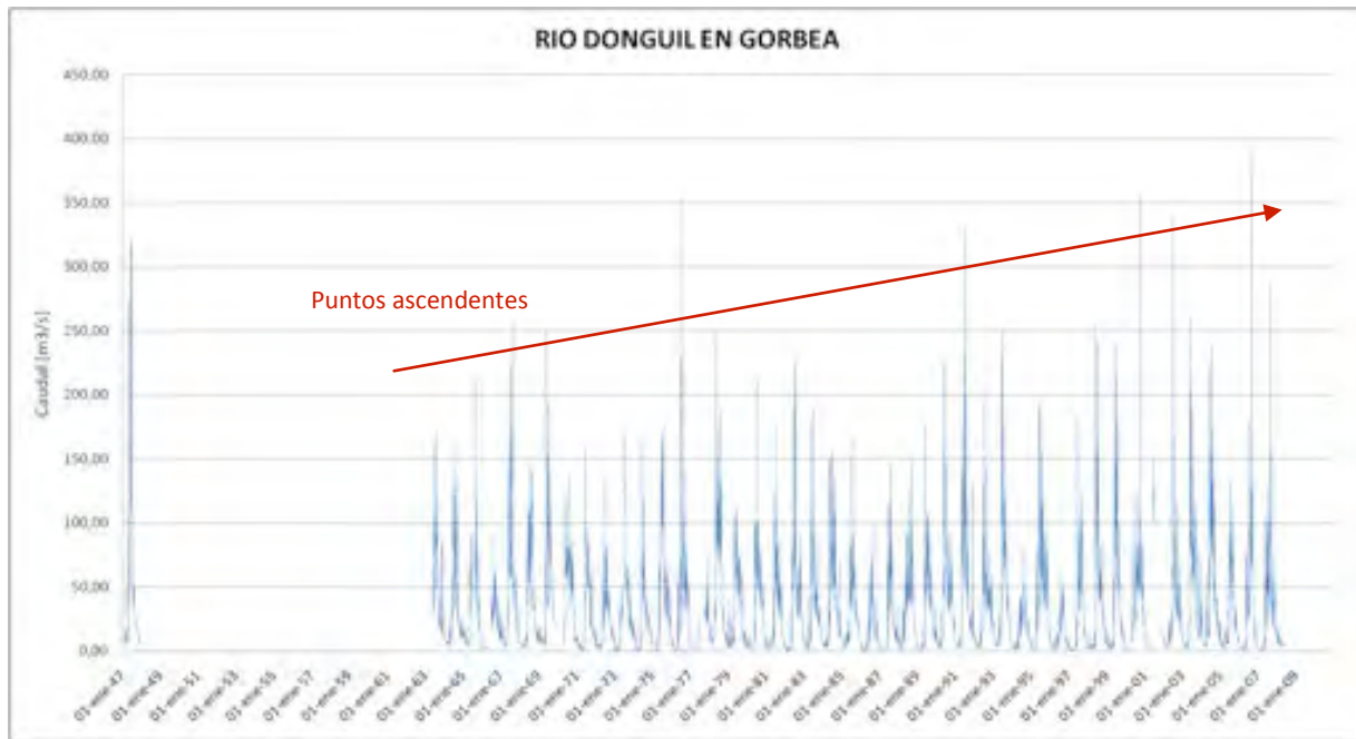
Ilustración 57: Caudales Río Dónguil - Puntos ascendentes
