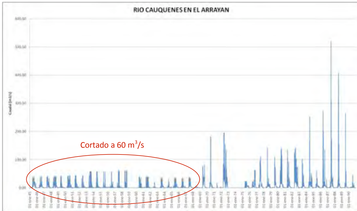
Ilustración 49: Caudales Río Cauquenes en el Arrayan – Años 1945-1969 malos
